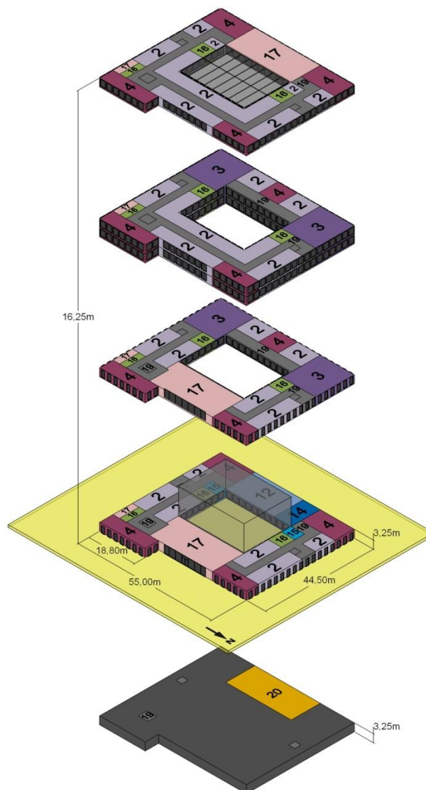
Bild 62: Büros - Module - Atrium - Darstellung Zonen - Ansicht Nord-Ost
