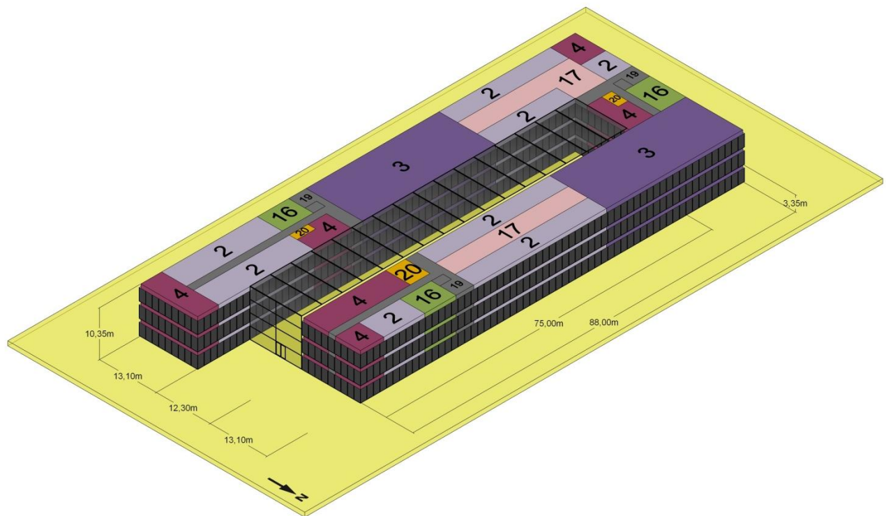
Bild 59: Büros - groß - Darstellung Zonen - Ansicht Nord-Ost
