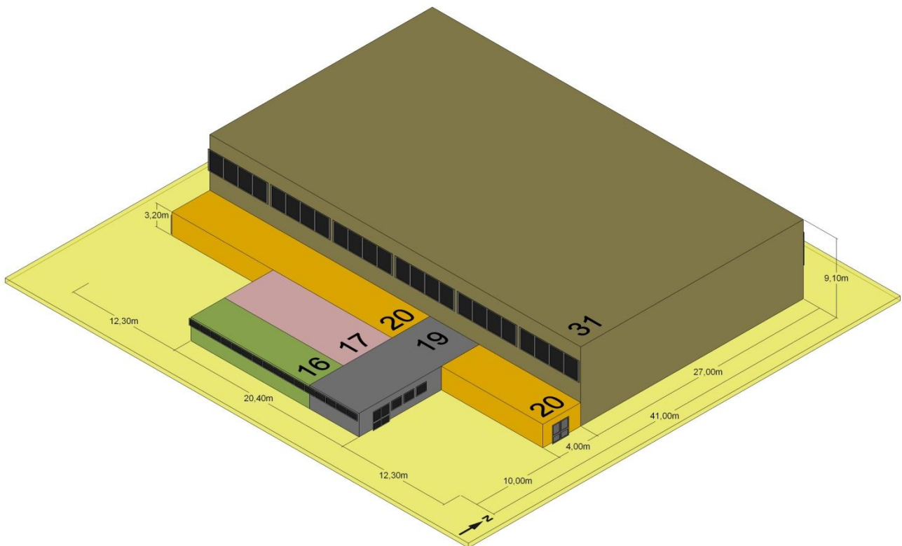
Bild 95: Dreifeld -Sporthalle – Darstellung Zonen – Ansicht Süd-Ost
